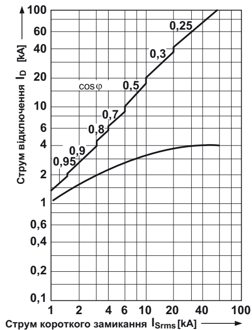
Струмо-обмежувача характеристика для M5P1
