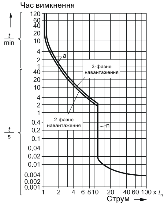
Струмо-часова характеристика для M5P1
