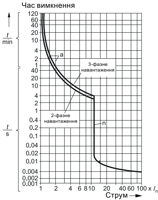
Струмо-часова характеристика для M5P0
