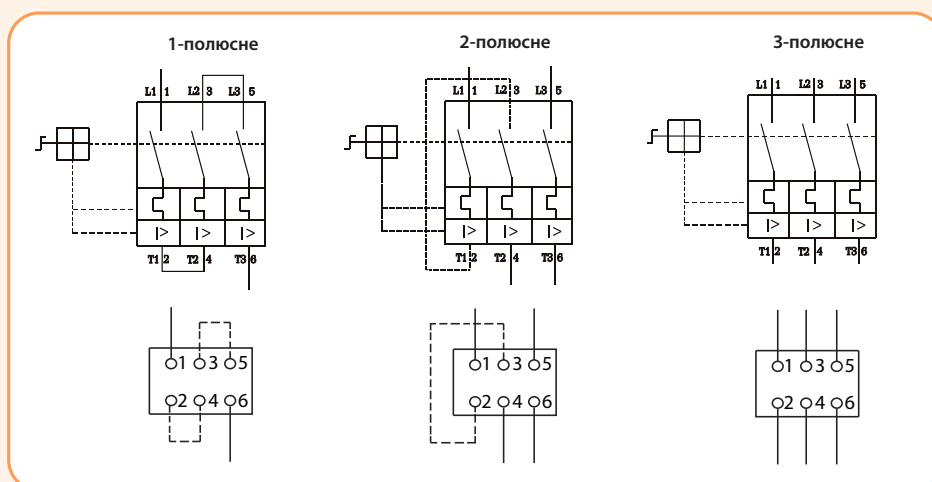
Схема підключення автоматичних вимикачів MS 25
