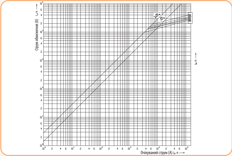
Характеристики обмеження струму ножових запобіжників NH2 400V із характеристикою gG
