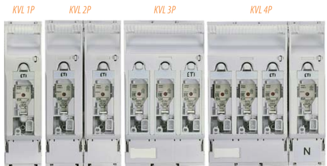
→ Горизонтальні роз'єднувачі запобіжників KVL доступні в 1-, 2-, 3-, 4-полюсному виконанні
