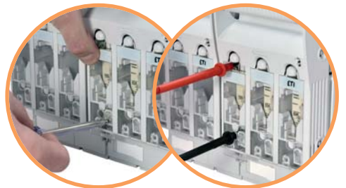
→ Зсувний захисний екран забезпечує доступ до зручного і безпечного проведення вимірювань
