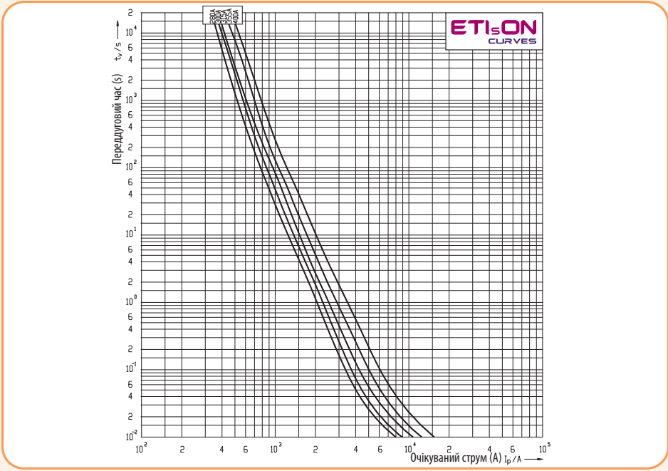
Характеристики обмеження струму ножових запобіжників NH2 400V із характеристикою gG
