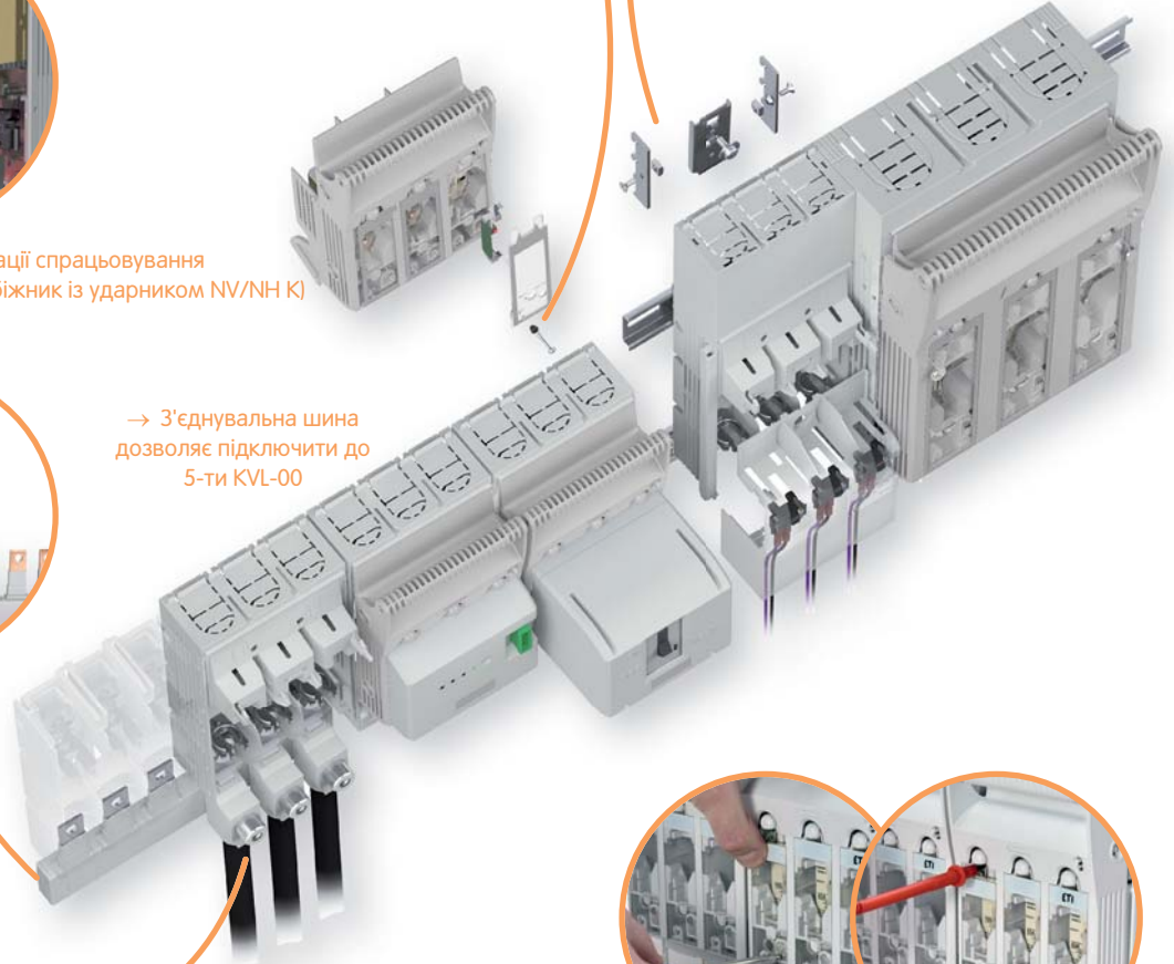
→ Роз'єднувачі KVL-00 та KVL-1 мають можливість монтажу на шину TH-35 за допомогою адаптера, а застосування довгих захисних кришок дозволяє встановлювати KVL-00 та KVL-1 в одну лінійку
